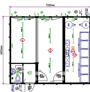
Kancelářské a sanitární kontejnery – trojitá sestava
