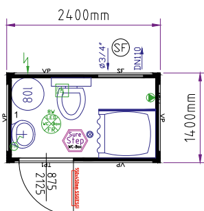
WC-kontejner se sprchou 8'
